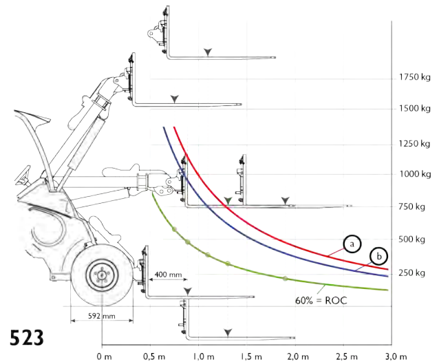
Diagramme de charge 523/528/530
